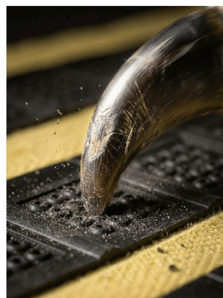
ツキノワグマの爪（現物）による強度テスト 炭素層はクマの爪が削れる硬度があります
